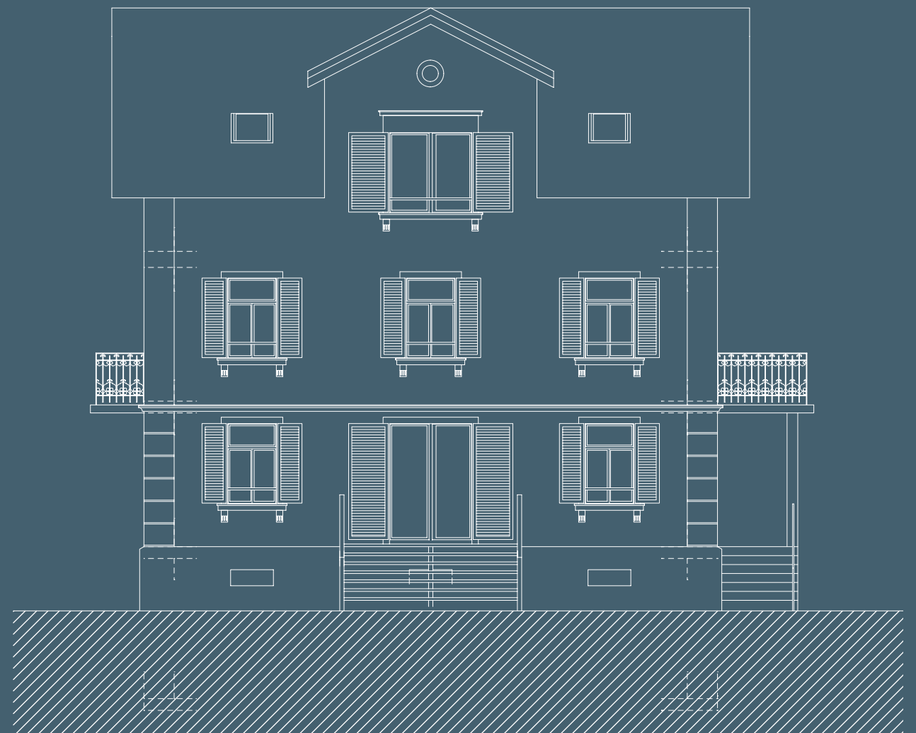
SÜD ANSICHT
