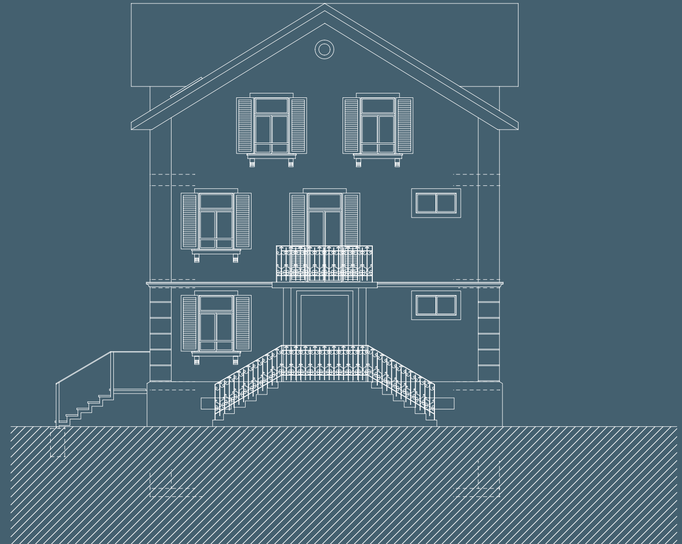
OST ANSICHT
